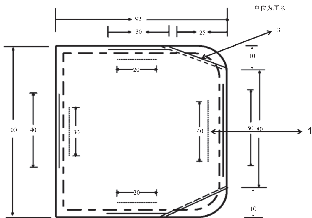
a) 小号羊衣平面展开图
