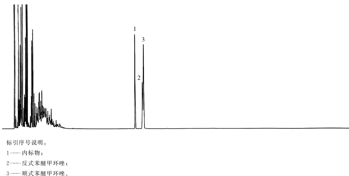
图 1 苯醚甲环唑微乳剂与内标物的气相色谱图
